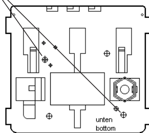
Porte-appareil pour fixation aux tubes
