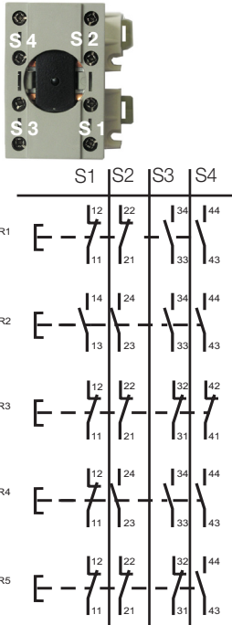
Drucktastersocket GHG41.11..R....; 2 x 2 polig
