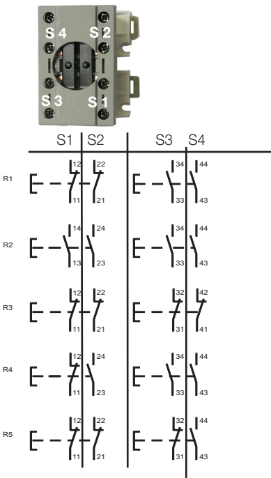
Kontaktbelegung
